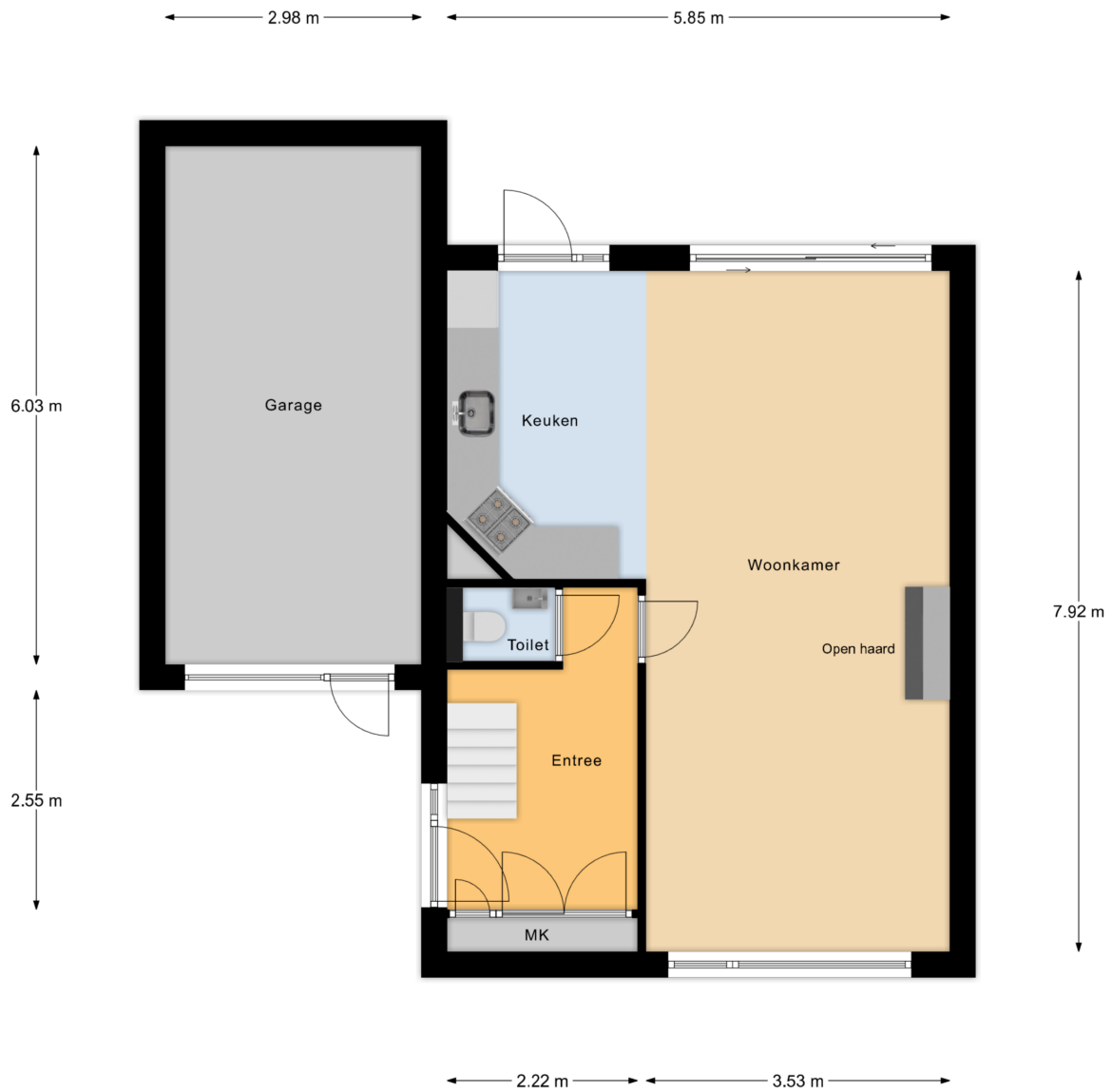
Begane Grond
