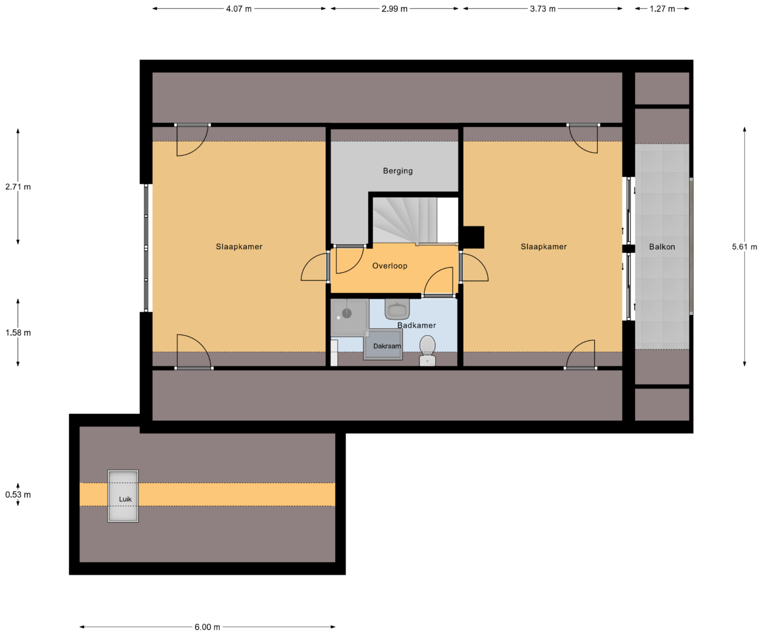
1e Verdieping
